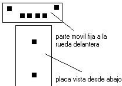
Figura 2. Sensores usados.
