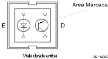
Figura 3.- El CNY70
